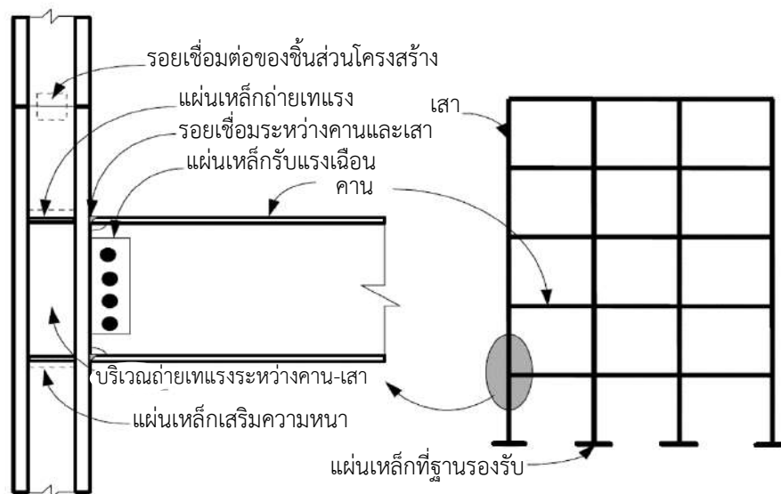
รูปที่ 17 ตำแหน่งที่มักจะได้รับความเสียหายของโครงสร้างเหล็กรับแรงดัด (ที่มา: FEMA-352)
